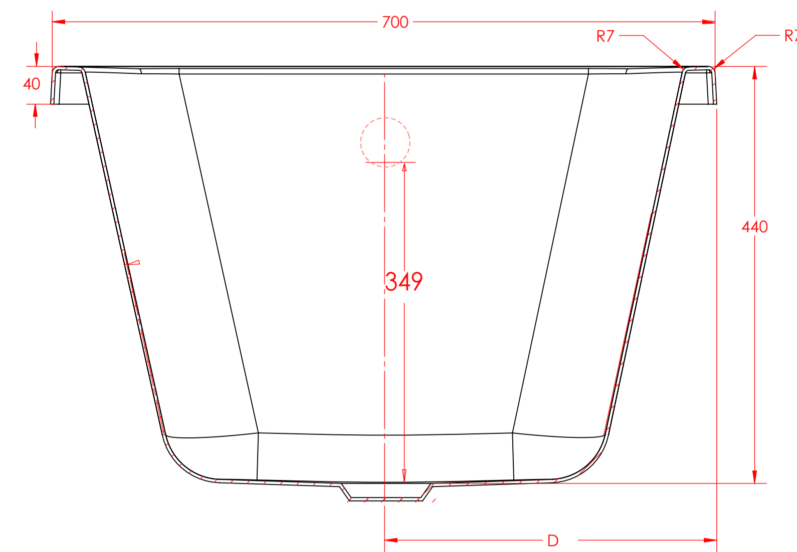
SECTION A-A SCALE 1 : 4
